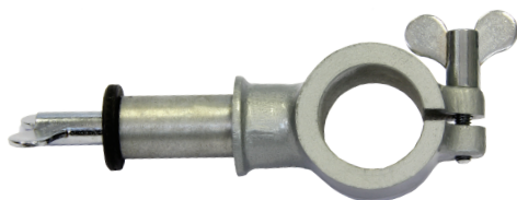
Suporte do Maçarico Oxyline C-205 para Autotrack 30/30A Ø 35mm sem cremalheira
