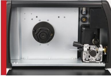
Alimentador de alambre interno
